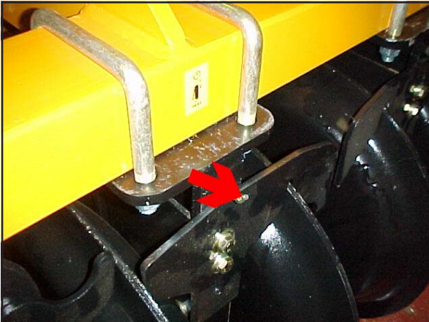
Fig. 5.01: DD Roll Grease Points
